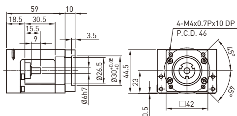
电机连接法兰 F2
