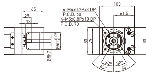
电机连接法兰F0
