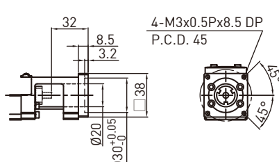
电机座F2
