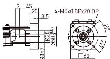
电机座F3
