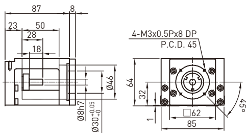
电机连接法兰 F3
