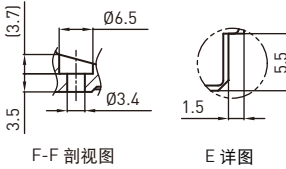
F-F 剖视图
