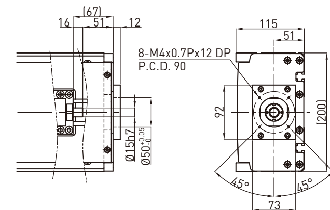
电机连接法兰F3
