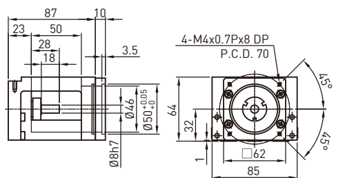
电机连接法兰
