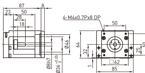
F1电机连接法兰 F5
