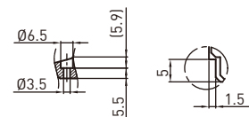
F-F 剖视图
