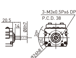
转接座H0
