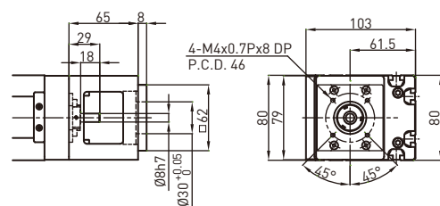
电机连接法兰F2
