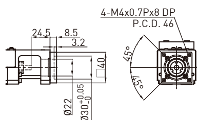
电机座F1
