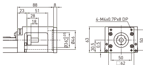
电机连接法兰 F5
