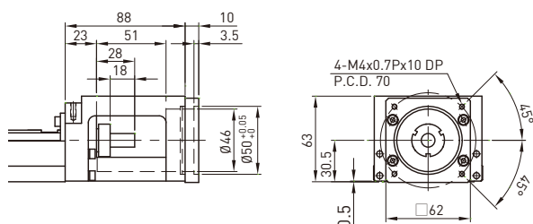
电机连接法兰 F2
