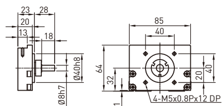
转接固定座 H0
