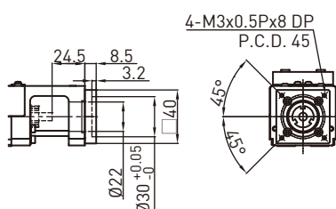
电机座F2
