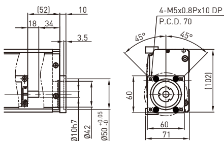
电机连接法兰F2
