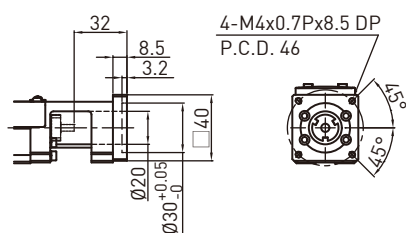
电机座F1
