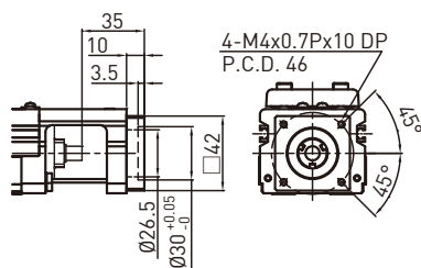
电机座F3
