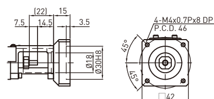
电机座F5
