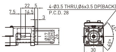
电机座F2
