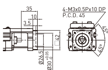
电机座F4
