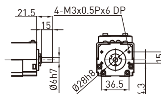
转接座H0
