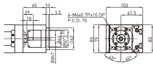
电机连接法兰F1
