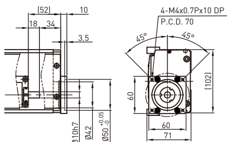
电机连接法兰F3
