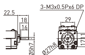
转接座H0
