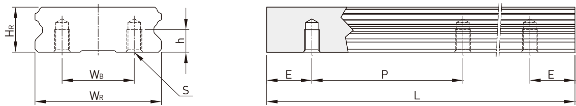
(3) WER-T下锁式导轨尺寸表
