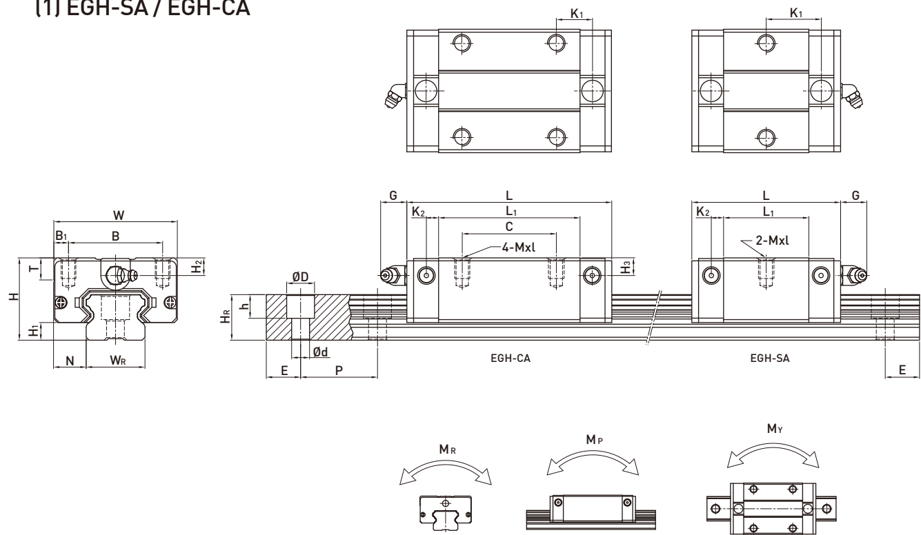
2-2-13 EG 系列直线导轨尺寸表
