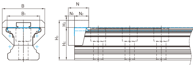
(6) CGR-CS 导轨防尘复盖带尺寸表
