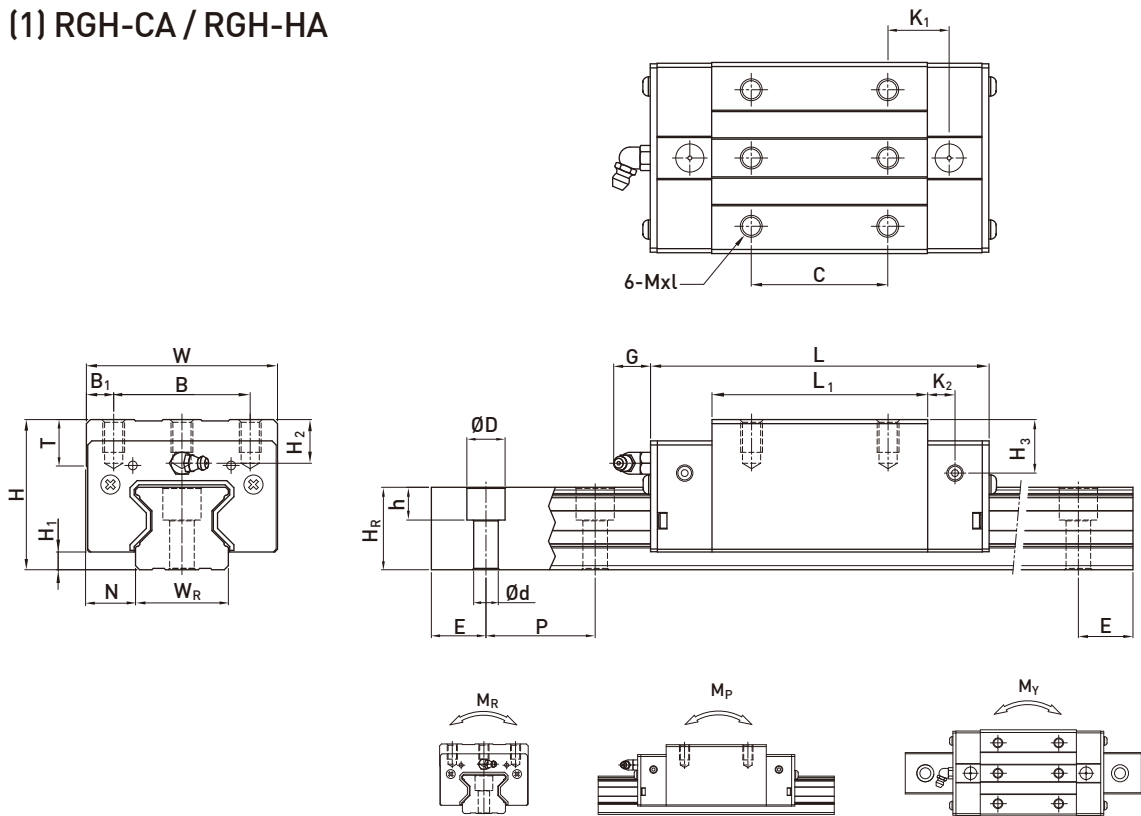
2-9-13 RG系列直线导轨尺寸表
