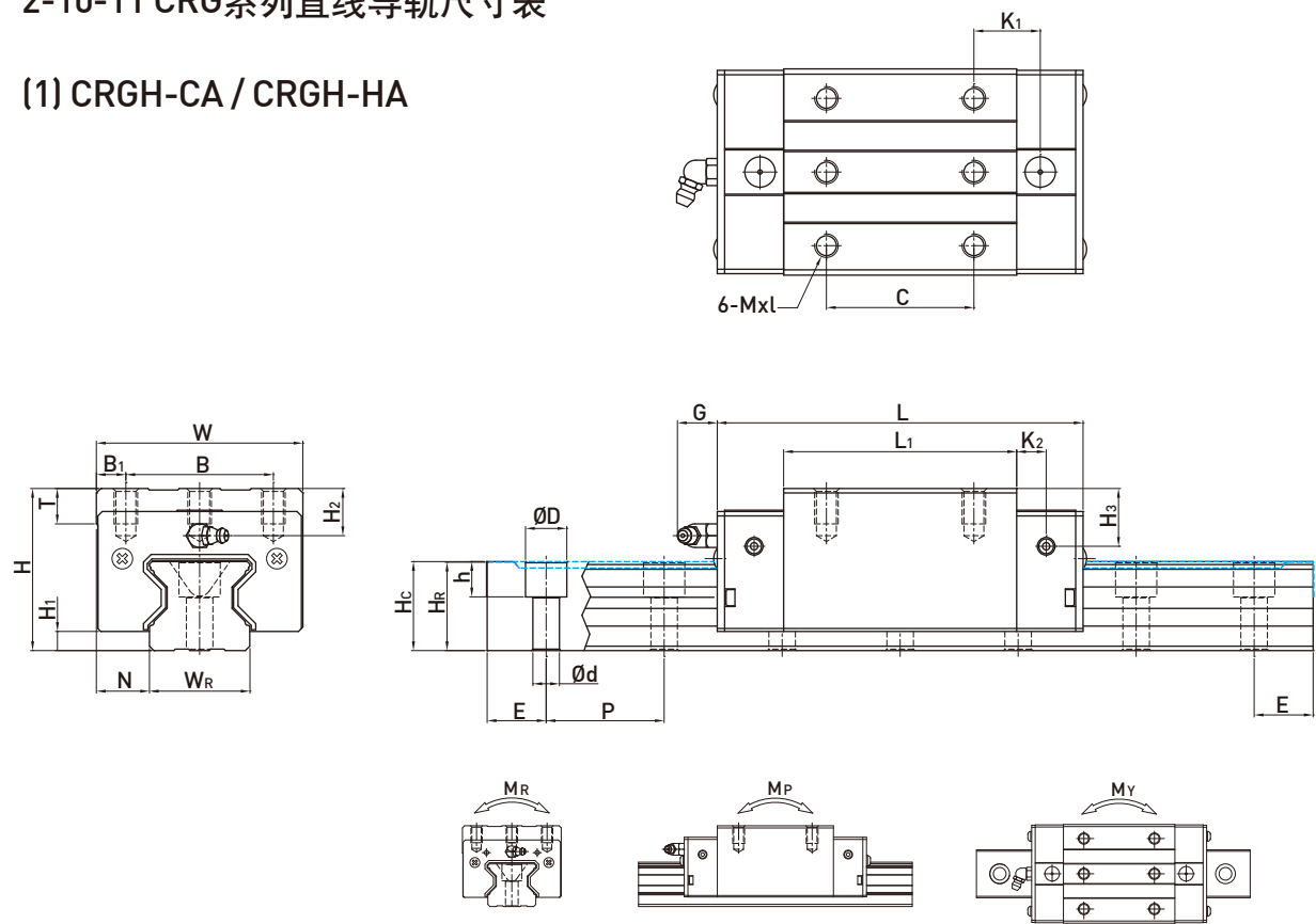
2-10-11 CRG系列直线导轨尺寸表
