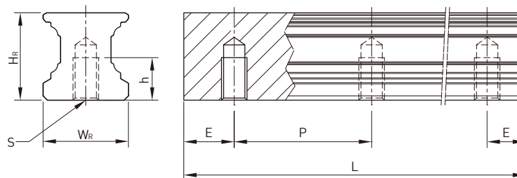
(5) CGR-T 下锁式导轨尺寸表
