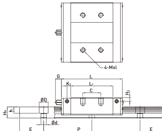
2-3-13 WE 系列直线导轨尺寸表
